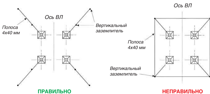
Рис. 1. Заземление опоры ВЛ
