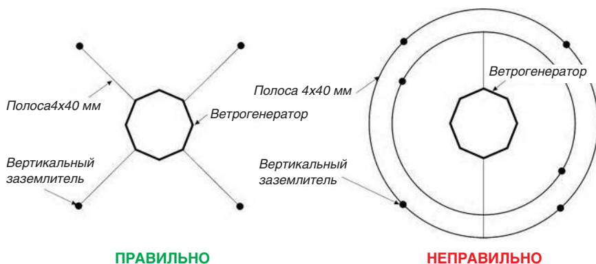
Рис. 2. Заземление ветрогенератора
