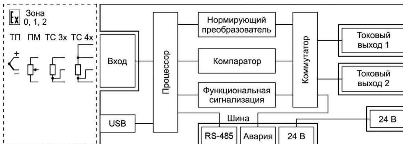
Рис. 1. Схема барьера искрозащиты KA5003Ex
