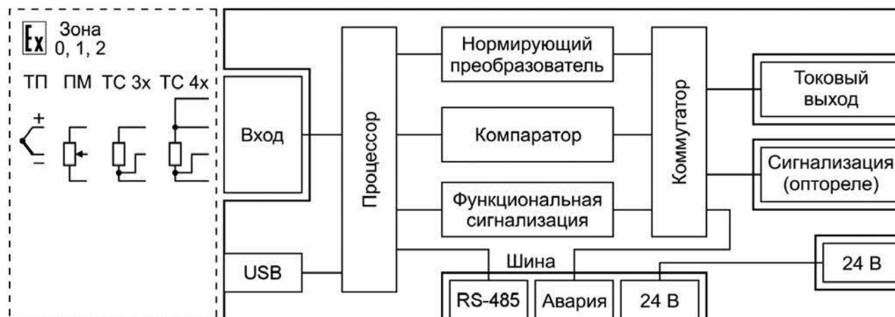
Рис. 2. Схема барьера искрозащиты KA5004Ex
