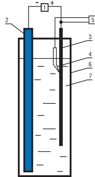
Рис. 3. Схема установки для испытания анодных заземлителей: 1 – источник постоянного тока 2 – катод (труба из нержавеющей стали) 3 – испытуемый анодный заземлитель 4 – хлор-серебряный электрод сравнения 5 – мультиметр APPA 103 N 6 – сосуд из полипропилена (100 л) 7 – испытательная среда (раствор NaCl 0,2 г/дм 3 )
