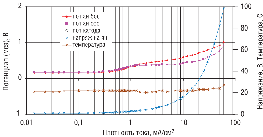
Рис. 2. Поляризационные кривые анода АЗК-ОП в глине естественной влажности (15–17%) с участка трассы действующего МГ
