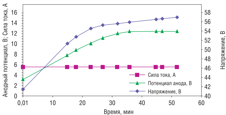
Рис. 5. Изменение анодного потенциала ТЭМС БТП во времени, достижение потенциала пробоя 12 В
