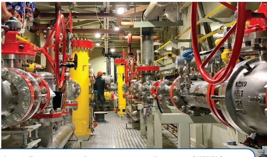
Фото 3. Технологический отсек газоприемной станции «ЭНЕРГАЗ»
